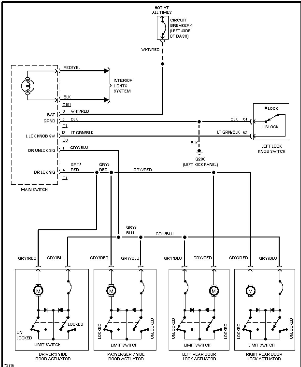
73716 Power Door Lock Circuit, Sedan
